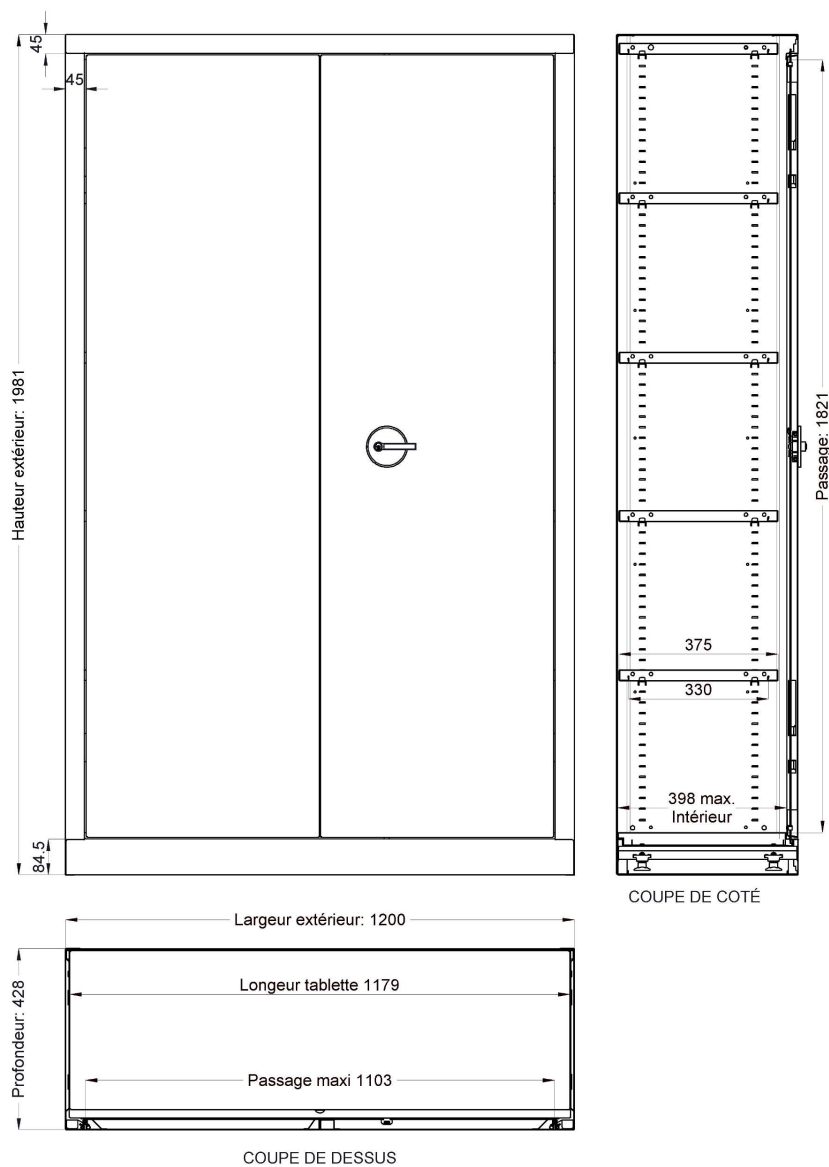
Géométraux de l'armoire PREMIUM portes battantes H.198 x L.120 x P.43cm
