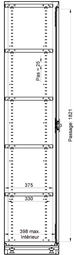
COUPE DE COTÉ
