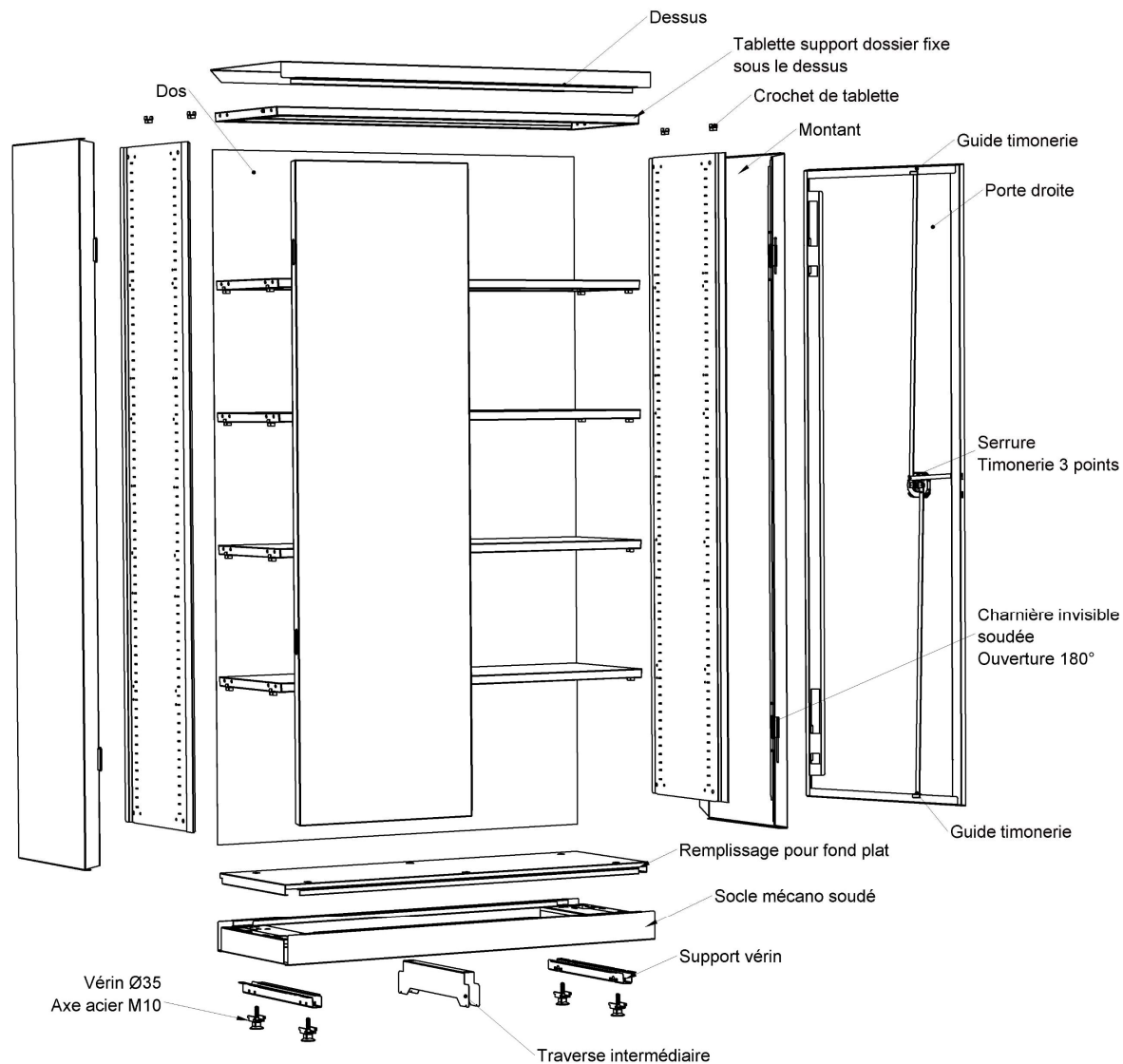
Eclaté de l'armoire PREMIUM portes battantes H.198 x L.120 x P.43cm
