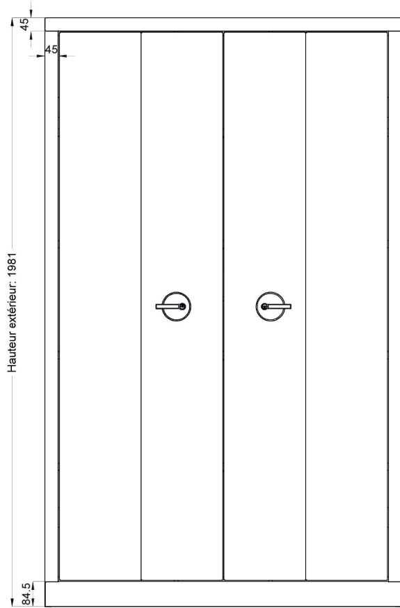
Géométraux de l'armoire PREMIUM portes pliantes H.198 x L.120 x P.43cm
