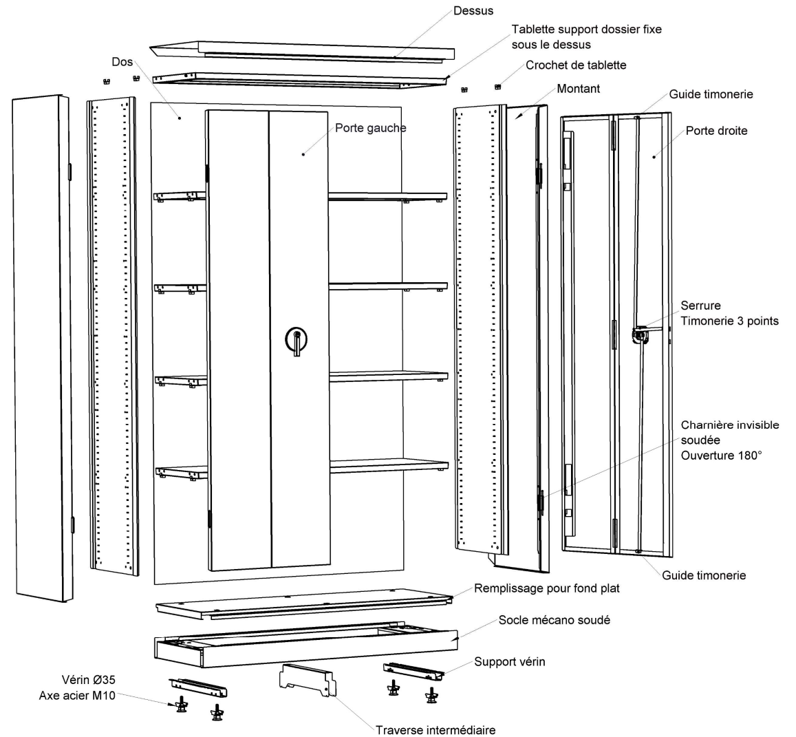
Eclaté de l'armoire PREMIUM portes pliantes H.198 x L.120 x P.43cm
